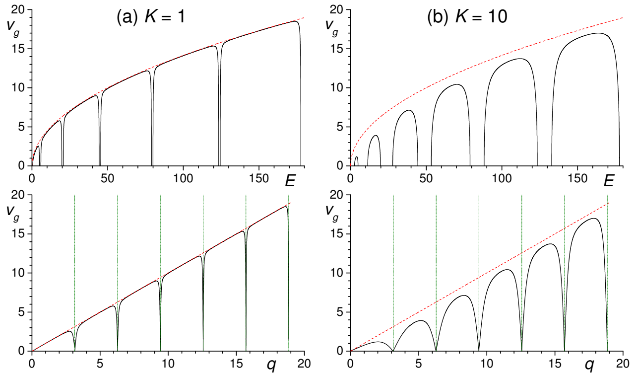
Obrázek 15: Grupová rychlost (7.4.4) v závislosti na energii (1. řádek) a na kvazihybnosti (2. řádek). Ve 2. řádku jsou hranice pásmů q = \pi n znázorněny svislými zelenými čerchovanými čarami. Červená čárkovaná čára odpovídá rychlosti pro volnou částici E = \hbar q/M .
