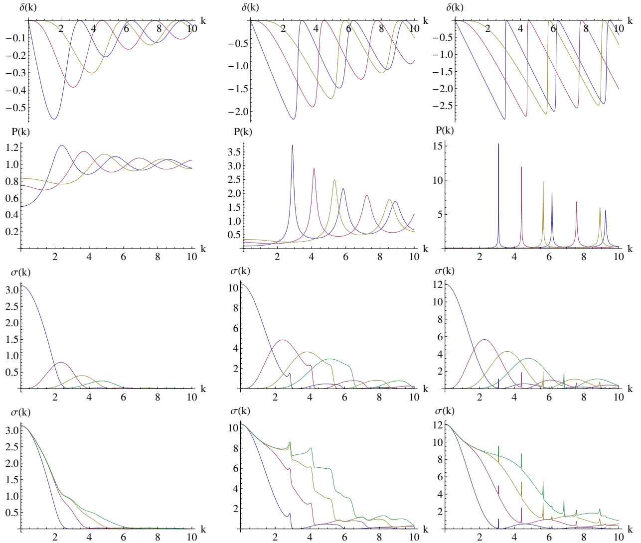
Obrázek 25: 1. řádek: Fázové posunutí l -té parciální vlny \delta_l(k) podle (15.4.14) pro l = 0 (modře), l = 1 (fialově), l = 2 (béžově). 2. řádek: Koefficient průniku l -té parciální vlny P_l(k) podle (15.4.15). 3. řádek: Účinný průřez l -té parciální vlny podle (15.4.18). 4. řádek: Součet účinných průřezů \sigma_0 (modře), \sigma_0 + \sigma_1 (fialově), \sigma_0 + \sigma_1 + \sigma_2 (béžově), \sigma_0 + \sigma_1 + \sigma_2 + \sigma_3 (zeleně). Vše je znázorněno pro různé hodnoty Q .
